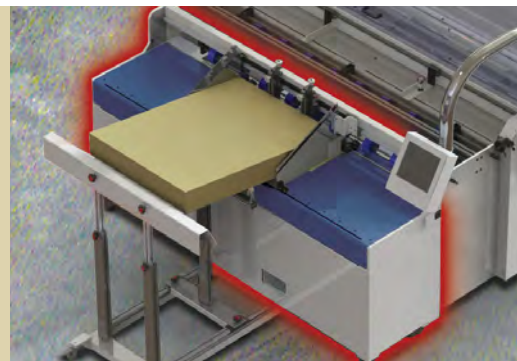
Anlegetisch für automatische Zuführung Einstellbar auf die gesamte Maschinenbreite
